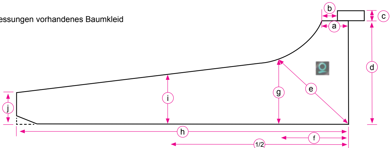
Aufmass an Bord
